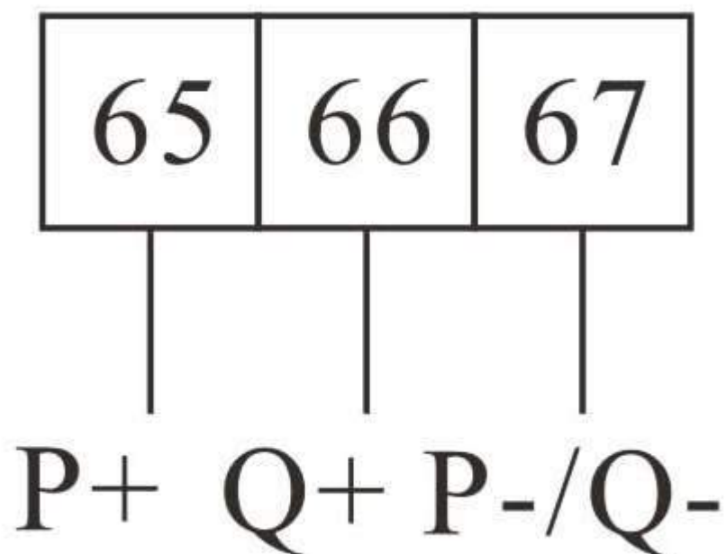
Рисунок 9. Импульсный выход
