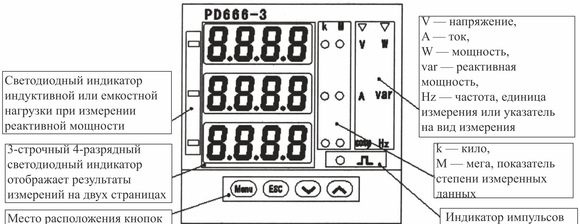
Рисунок 24. Изображение панели
