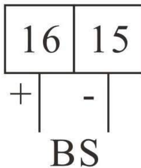
Рисунок 7. Сигнальный выход
