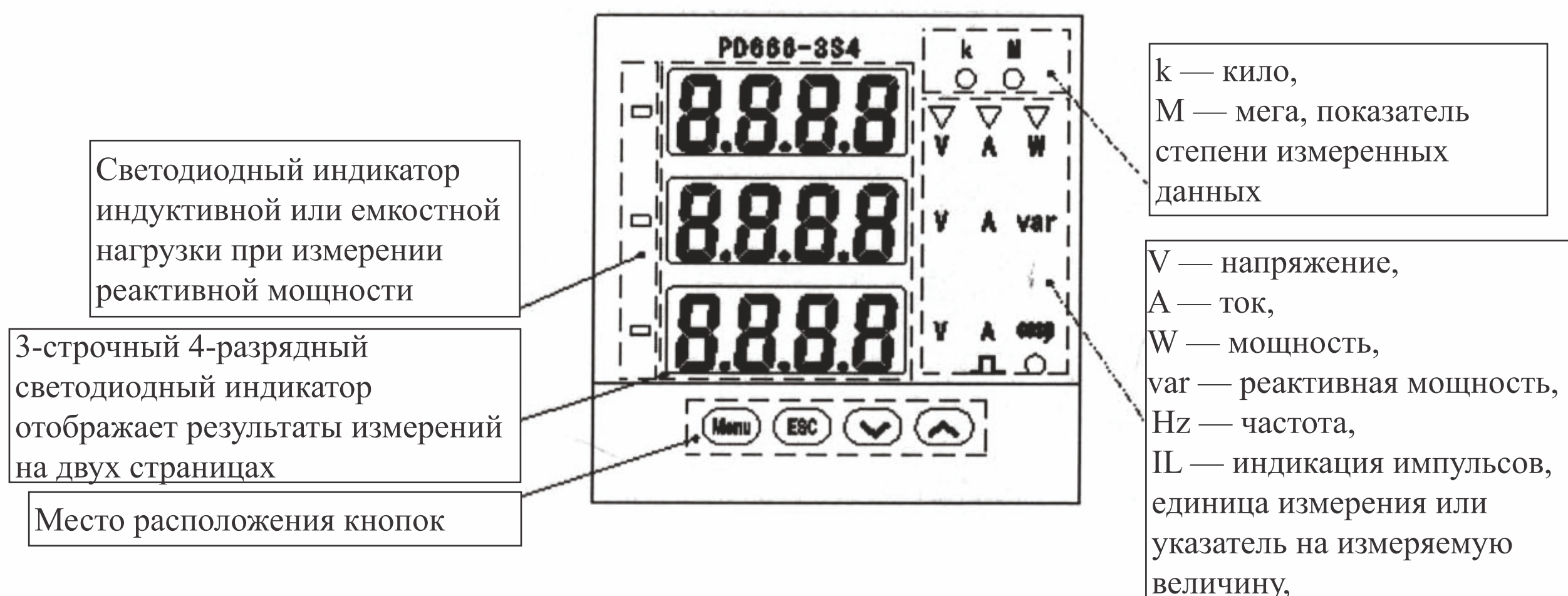
Рисунок 26. Изображение панели
